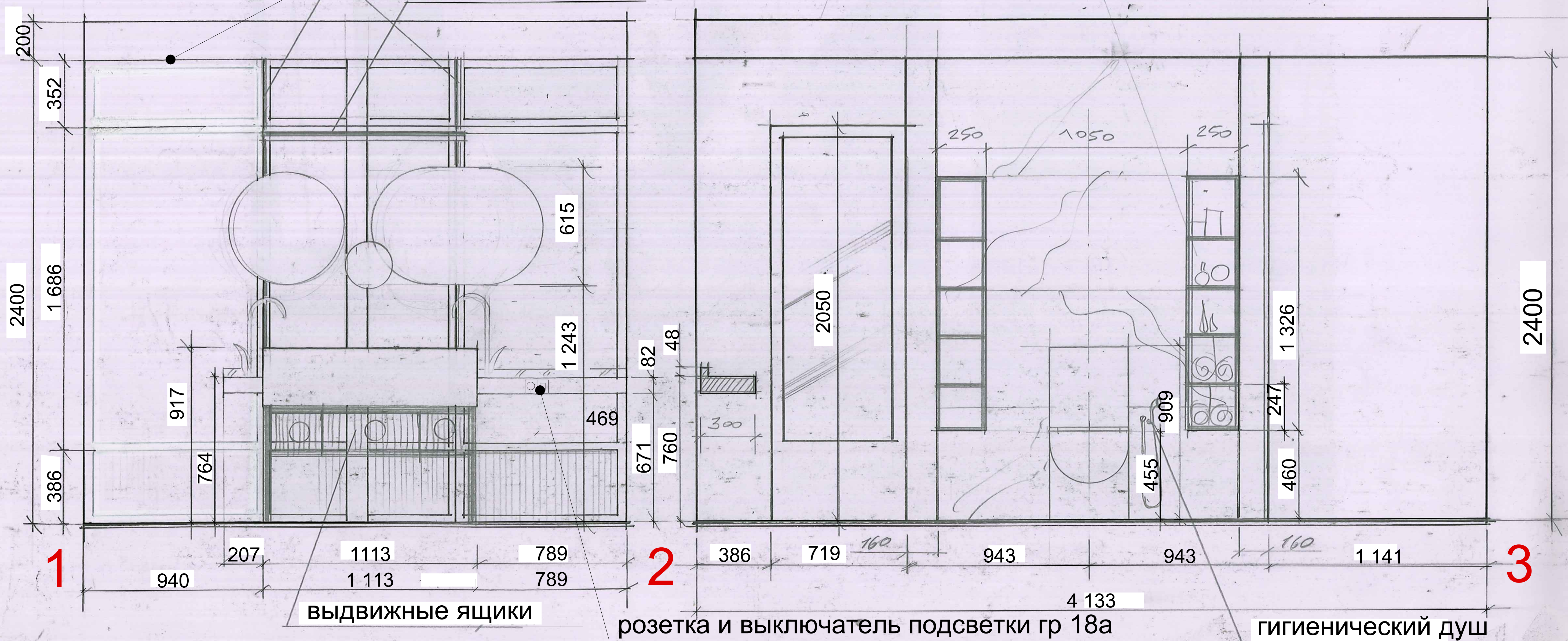
подвесной потолок крепление зеркал подсветка Н=2000мм
