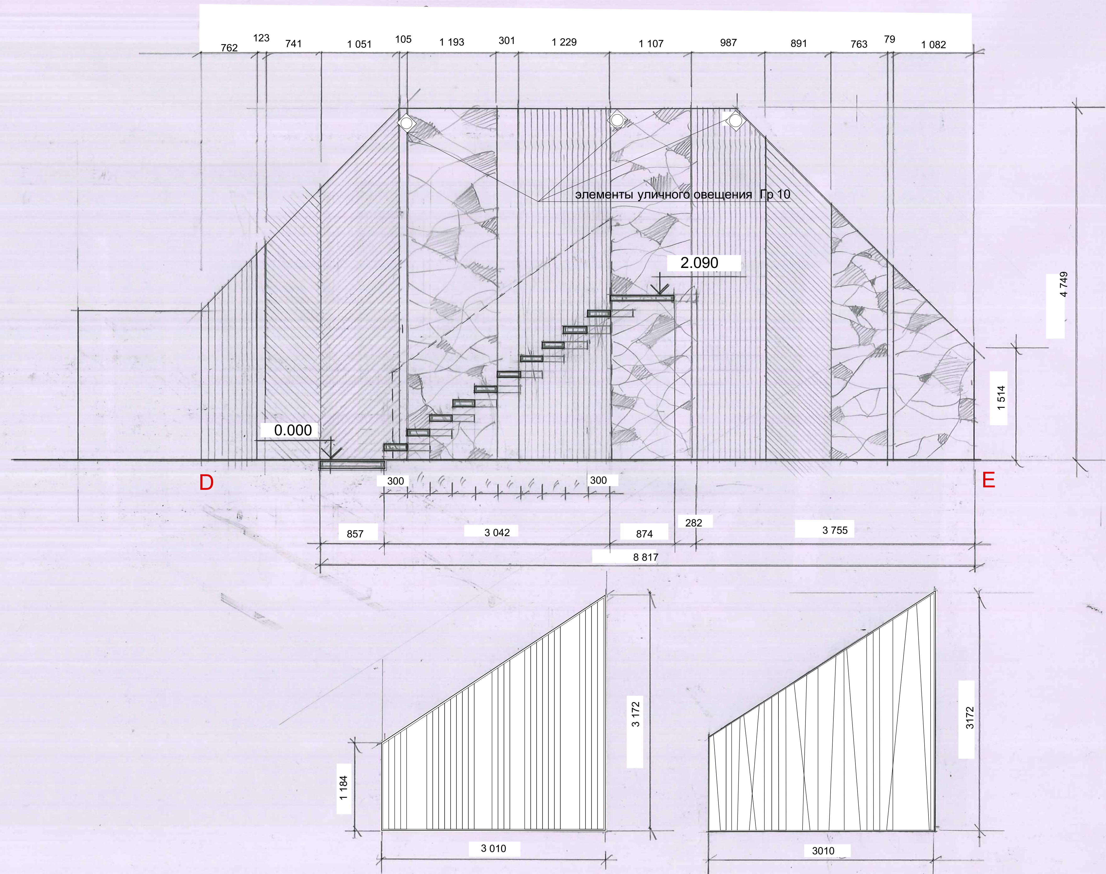
Варианты ограждения лестницы М 1:50
