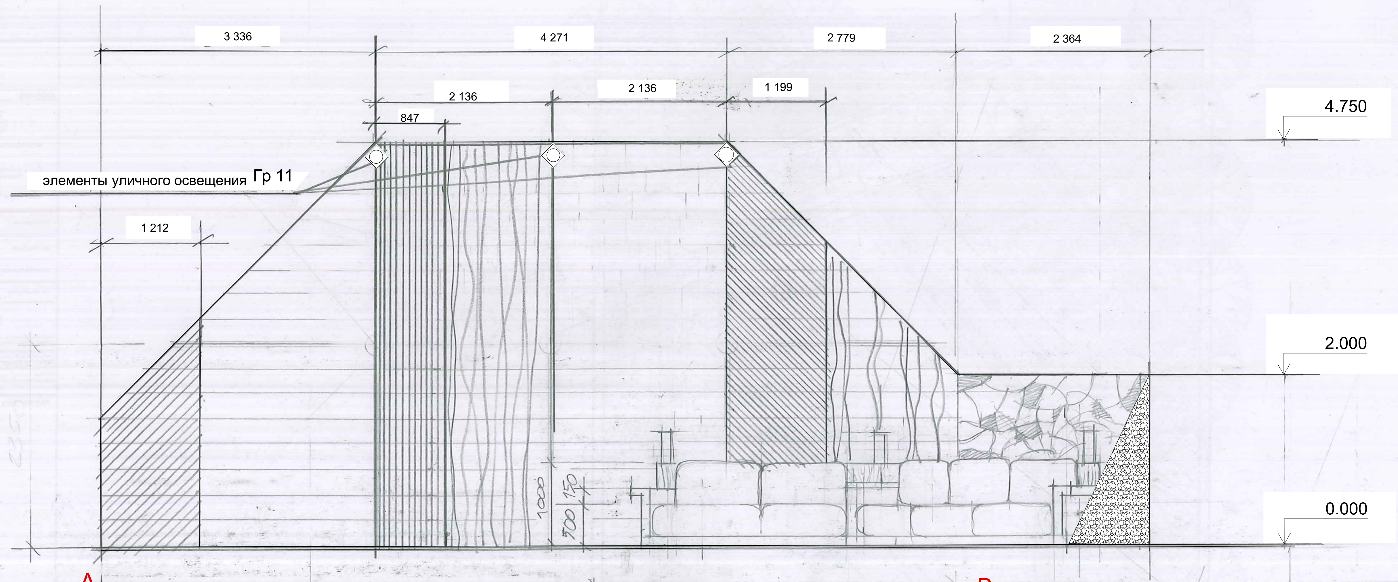
Расвертка стены участка А,В,С М 1:50
